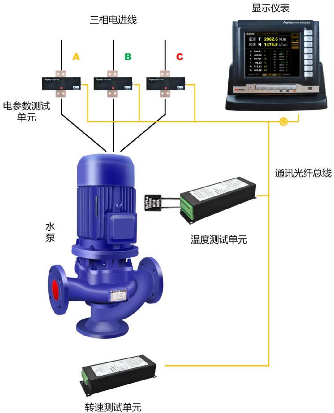
图2 TN4000 电子式扭矩仪构成原理
